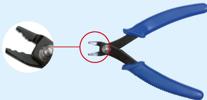
Art. NC22 – Quetschzange für Metallperlen, speziell geformte Backenprofile Item NC22 – Crimping pliers for metal beads, specially shaped jaw profiles
